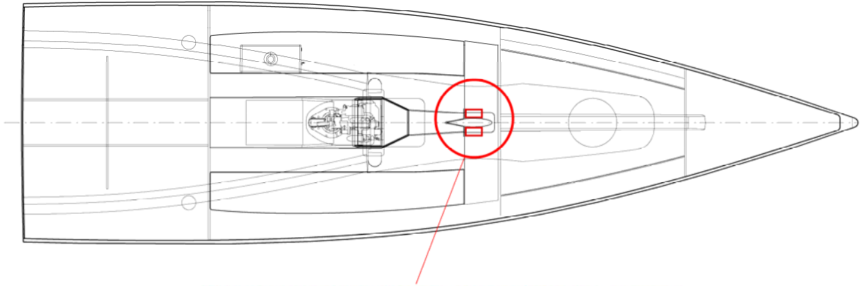
Position longitudinale et transversale des poids correcteurs
